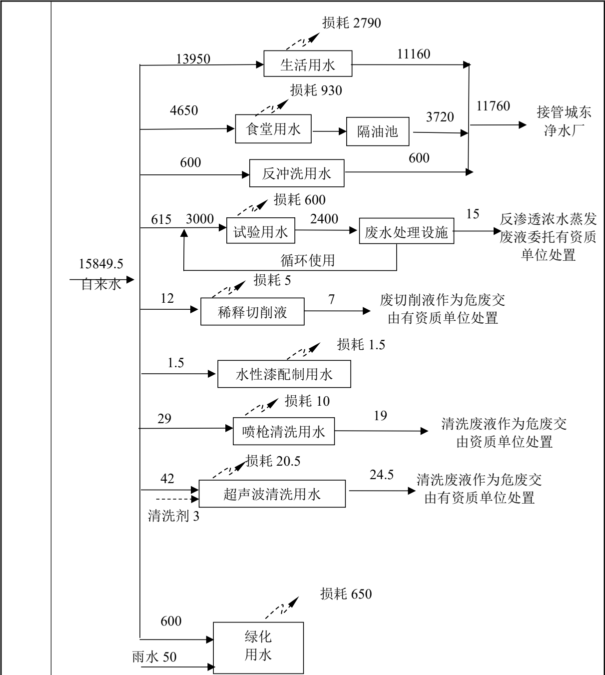
图2-2全厂水平衡图 单位：t/a
