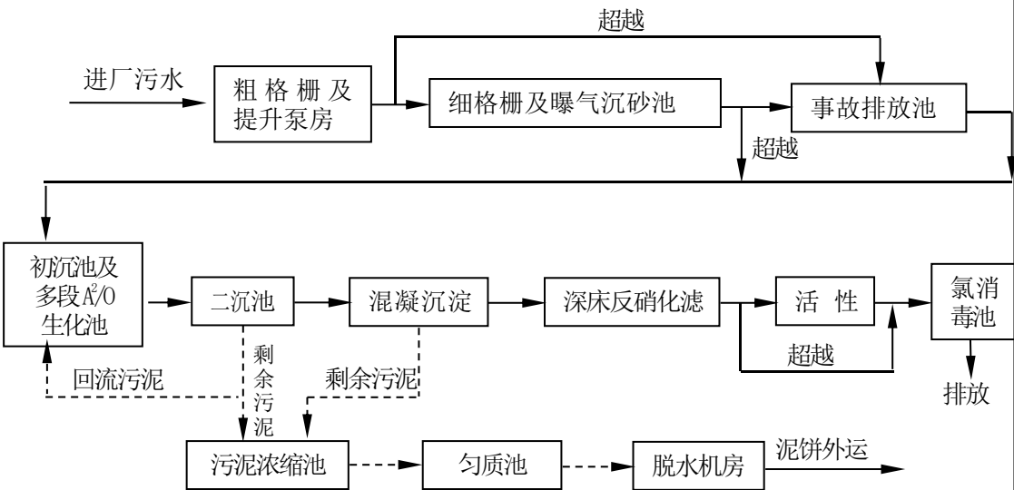
图 4-2 江苏中法水务股份有限公司（城东水质净化厂）废水处理工艺流程图 根据对城东水质净化厂工业废水污染源的调查，工业废水、生活污水的水质推测，通过生活污水量和工业废水量的比例，并结合区域的实际水质情况，城东水质净化厂尾水排放执行江苏中法水务股份有限公司（城东水质净化厂）环境影响评价报告表、环评批复及《关于准予常熟市城东水质净化厂在大翁新建入河排污口的行政许可决定》（常熟市水利局行政许可决定书常水许可〔2018〕46 号）的相关要求，见下表。
